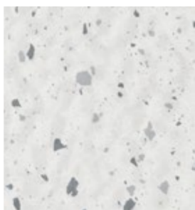
S 101
