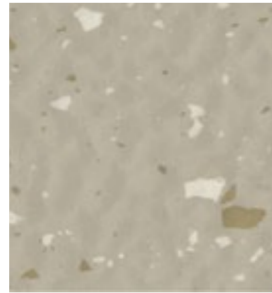
S 111
