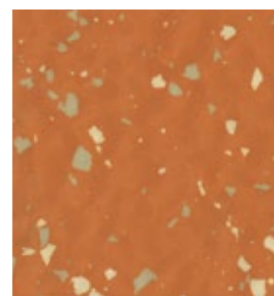
S 118
