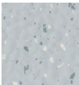
S 107
