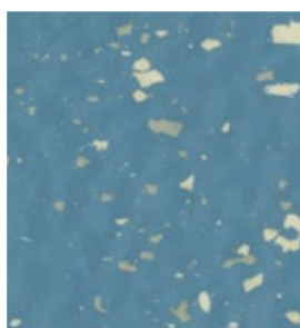
S 115
