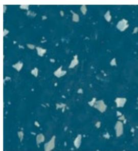
S 121
