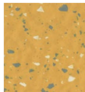
S 112
