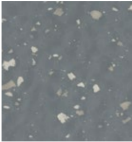
S 116
