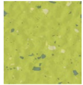
S 103
