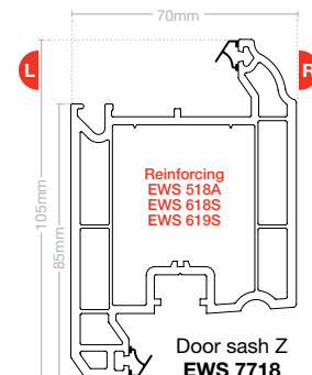
Door sash Z EWS 7718
